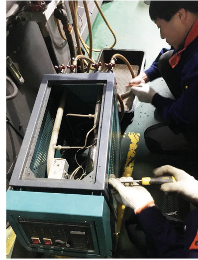
安装沃肯(Vulcan)一年半后 拆开模温机检查换热器
